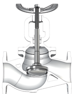
С регулирующим затвором
