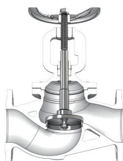
С балансировочным затвором
